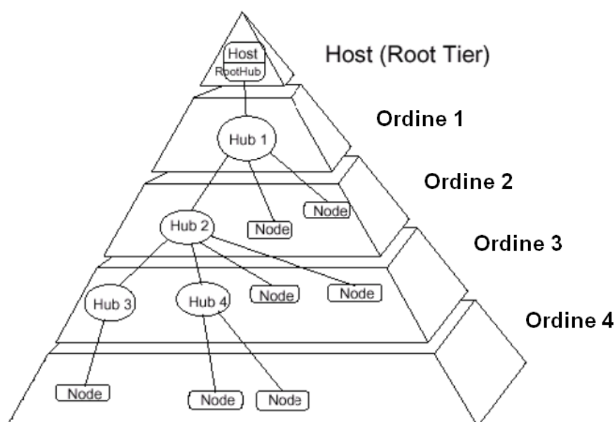
Fig. 2 - Schema di connessione tra periferiche e HUB.
