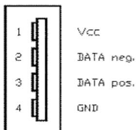
Connettore USB (lato innesto)
