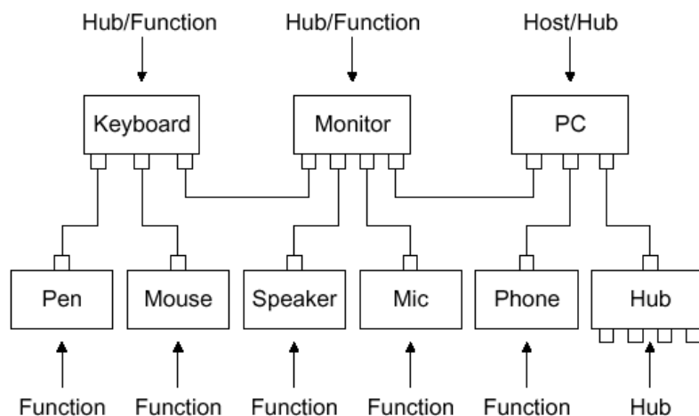
Fig. 2 - Schema di connessione tra periferiche e HUB.
