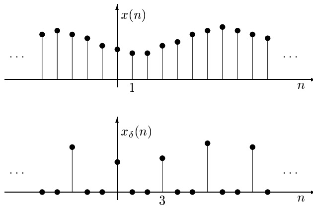
Figura 3.23: Il campionamento ideale di una sequenza.
