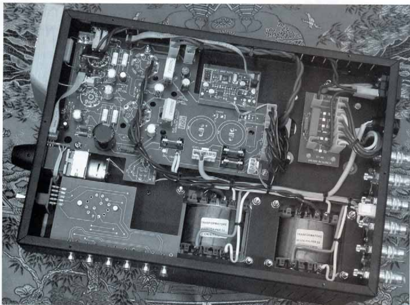
△ 15週年紀念限量版Simply Two的內部結構，兩隻輸出牛是特製新品。
