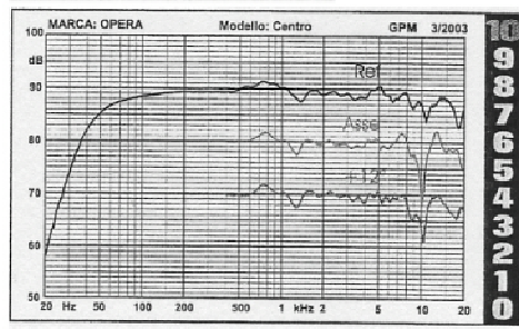
Risposta a varie angolazioni verticali
