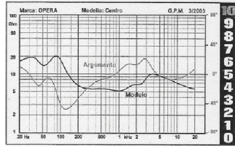
Modulo ed argomento dell'impedenza
