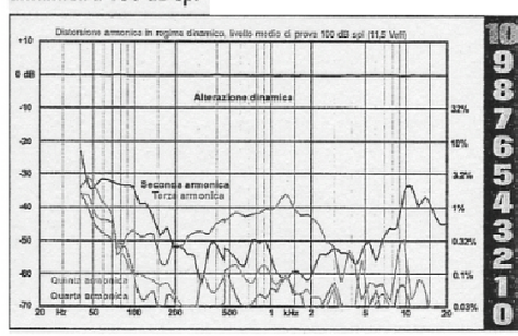
Distorsione di 2°, 3°, 4°, 5° armonica ed alterazione dinamica a 100 dB SPL
