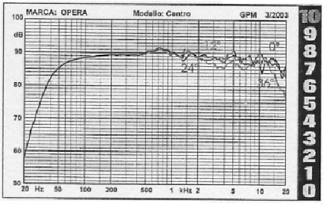
Risposta a varie angolazioni orizzontali
